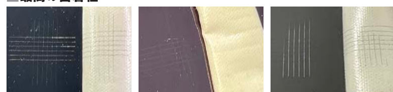
●スレート ●ガルバリウム ●ガラス ■試験方法/①各基材に弊社塗料を直接塗装②乾燥後塗膜にクロスカット(基準目試験)③強力ガムテープを貼り付け、剥がす
